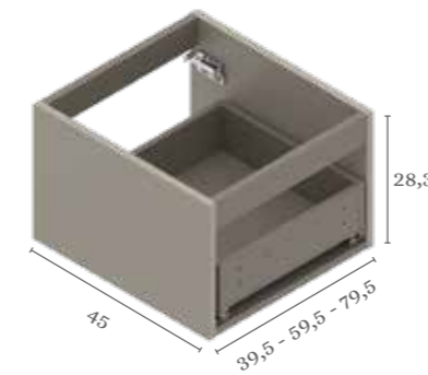
Mobile basso 1 cassetto / mobile basso 2 cassetti
