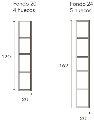
Alto abierto
