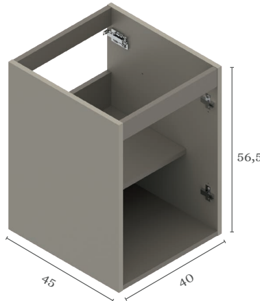
Bajo 1 puerta
