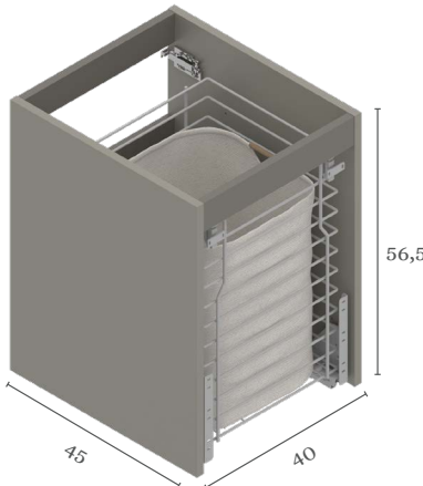
Bajo ropero
