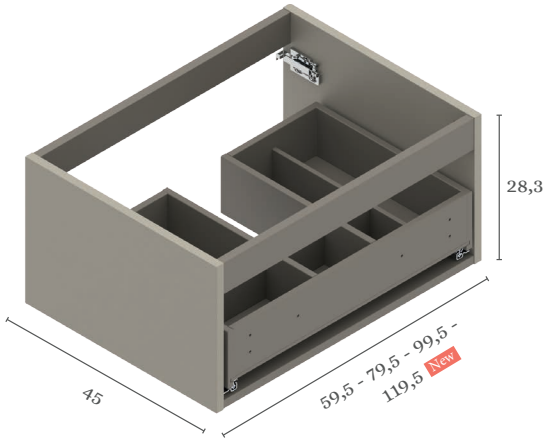
Mueble 1 cajón
