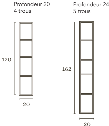
Meuble haut ouvert
