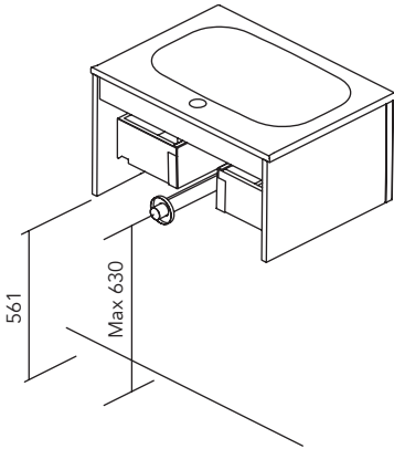
1 tiroir. Profondeur vide sanitaire 7 cm.
