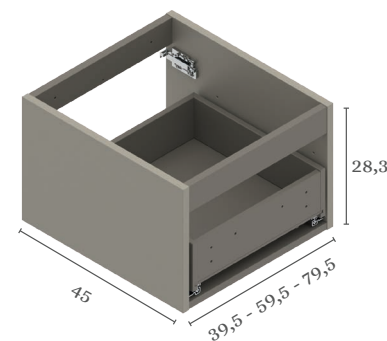
Meuble bas 1 tiroir / Meuble bas 2 tiroirs
