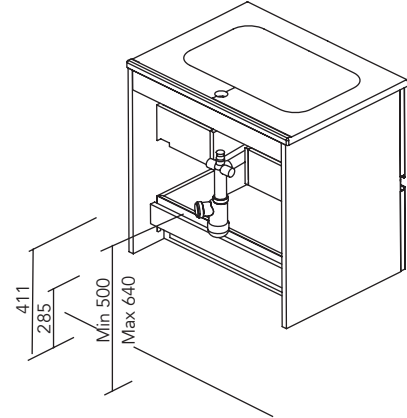
2 tiroirs. Profondeur vide sanitaire 7 cm.
